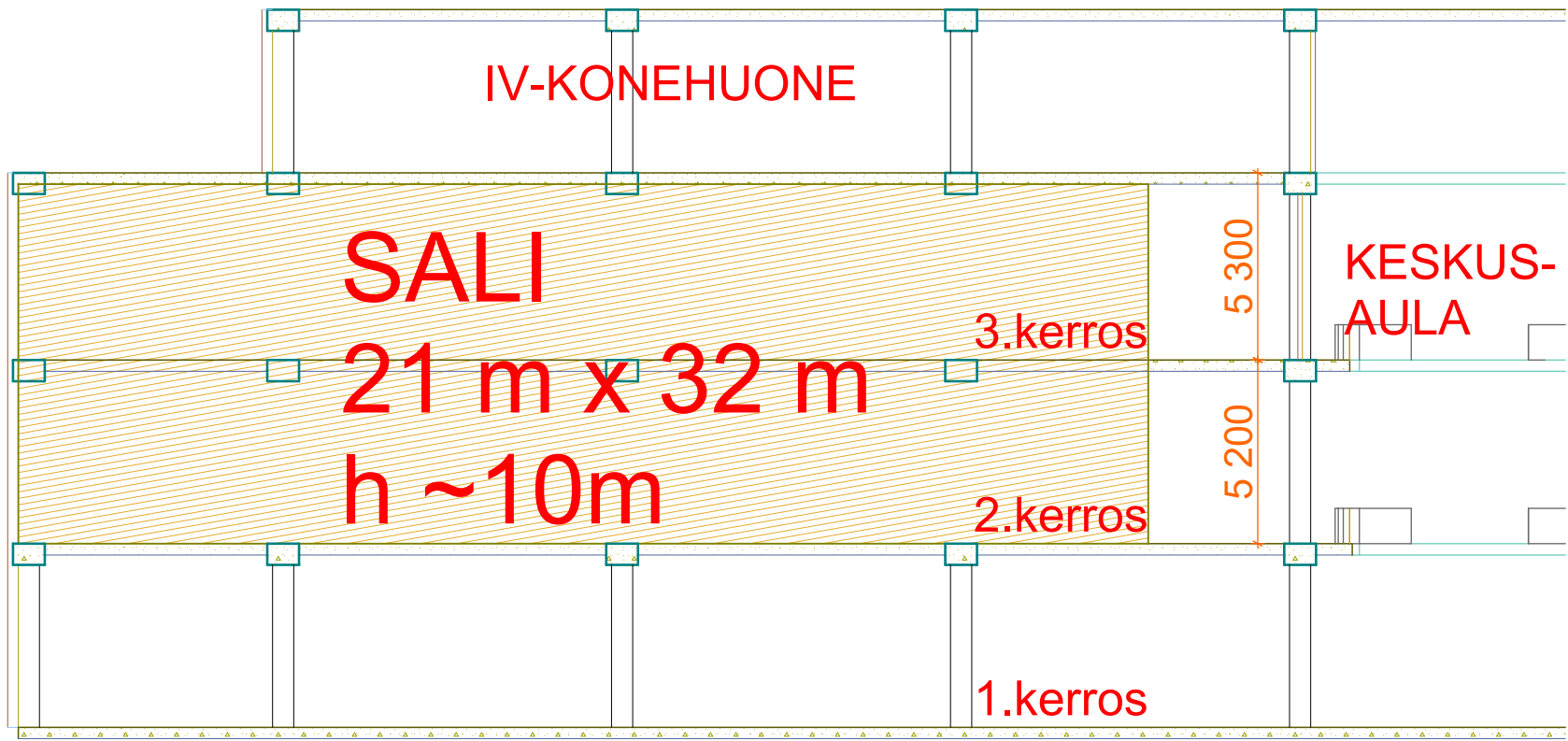
Leikkaus B - B 1 : 2 0 0
