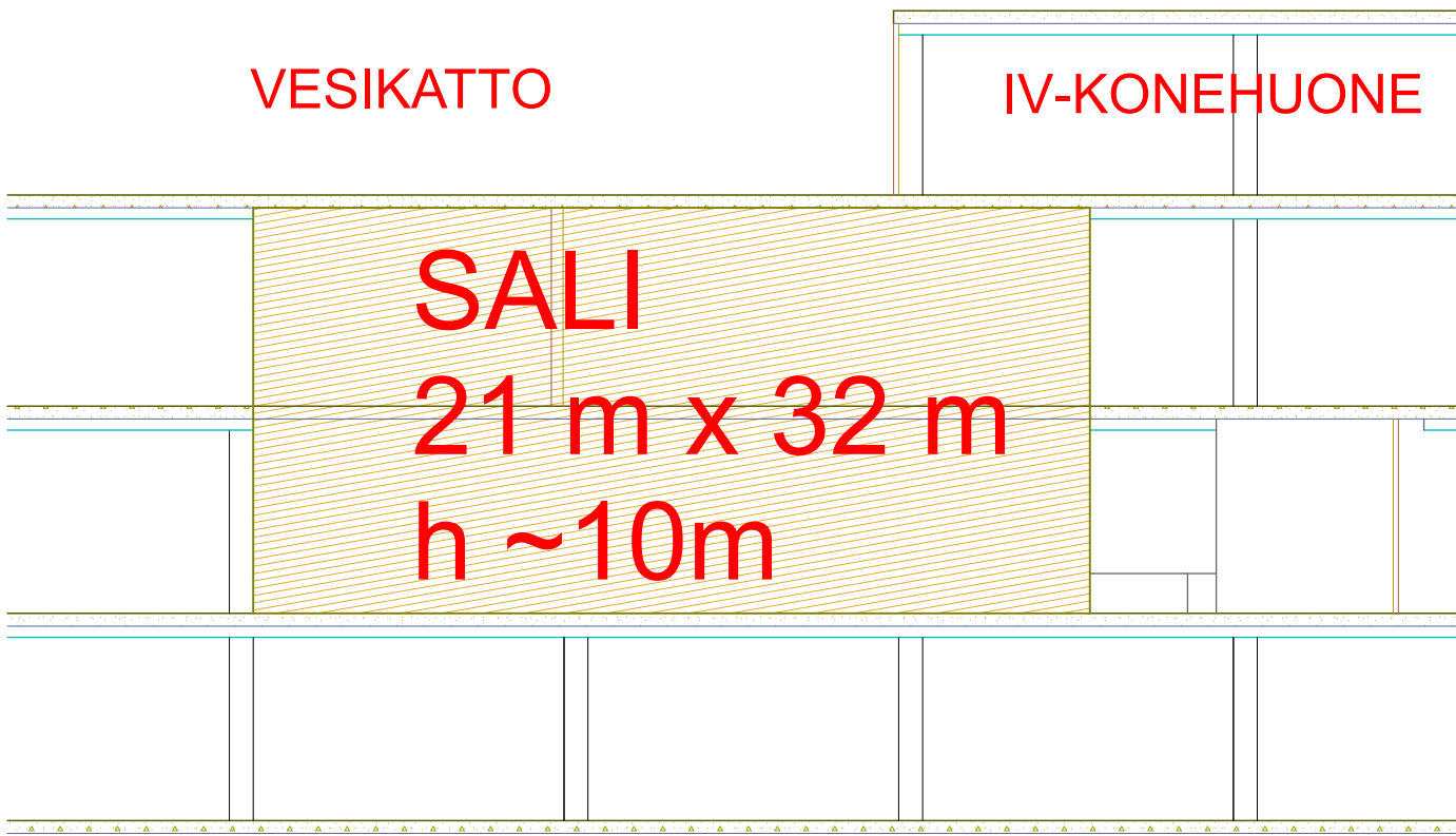
Leikkaus A - A 1 : 2 0 0
